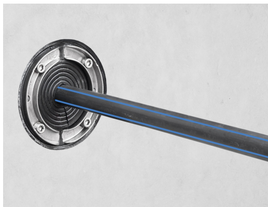
Vodovodné potrubie utesnené tesnením HSD 100 SSG 18-65
